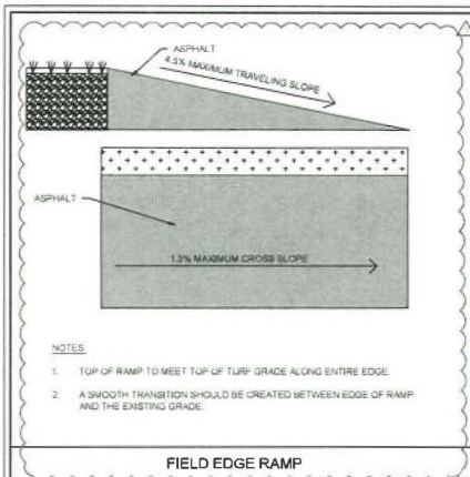
FIELD EDGE RAMP
