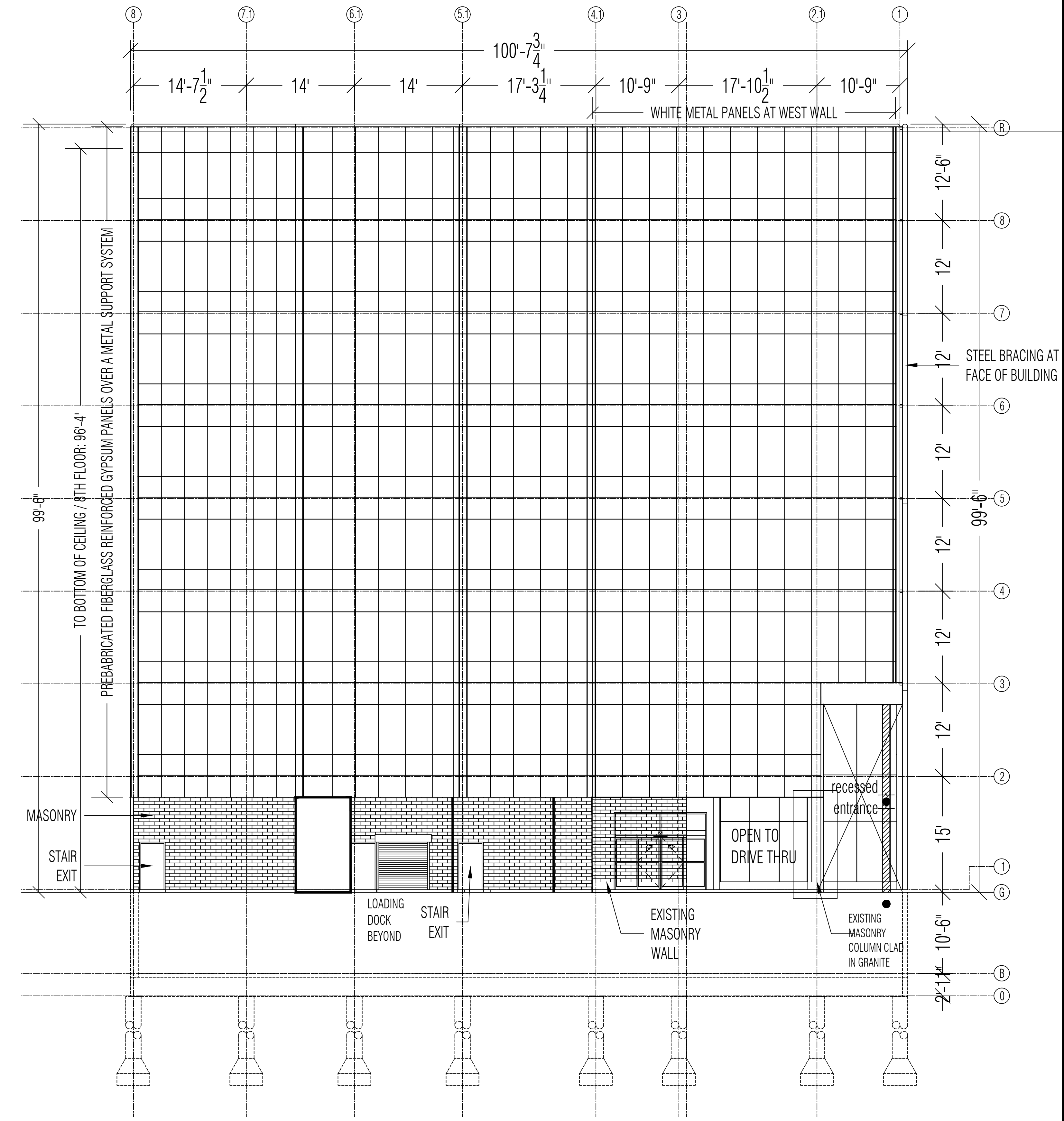
2 WEST ELEVATION Scale: 1/8" = 1'-0"
