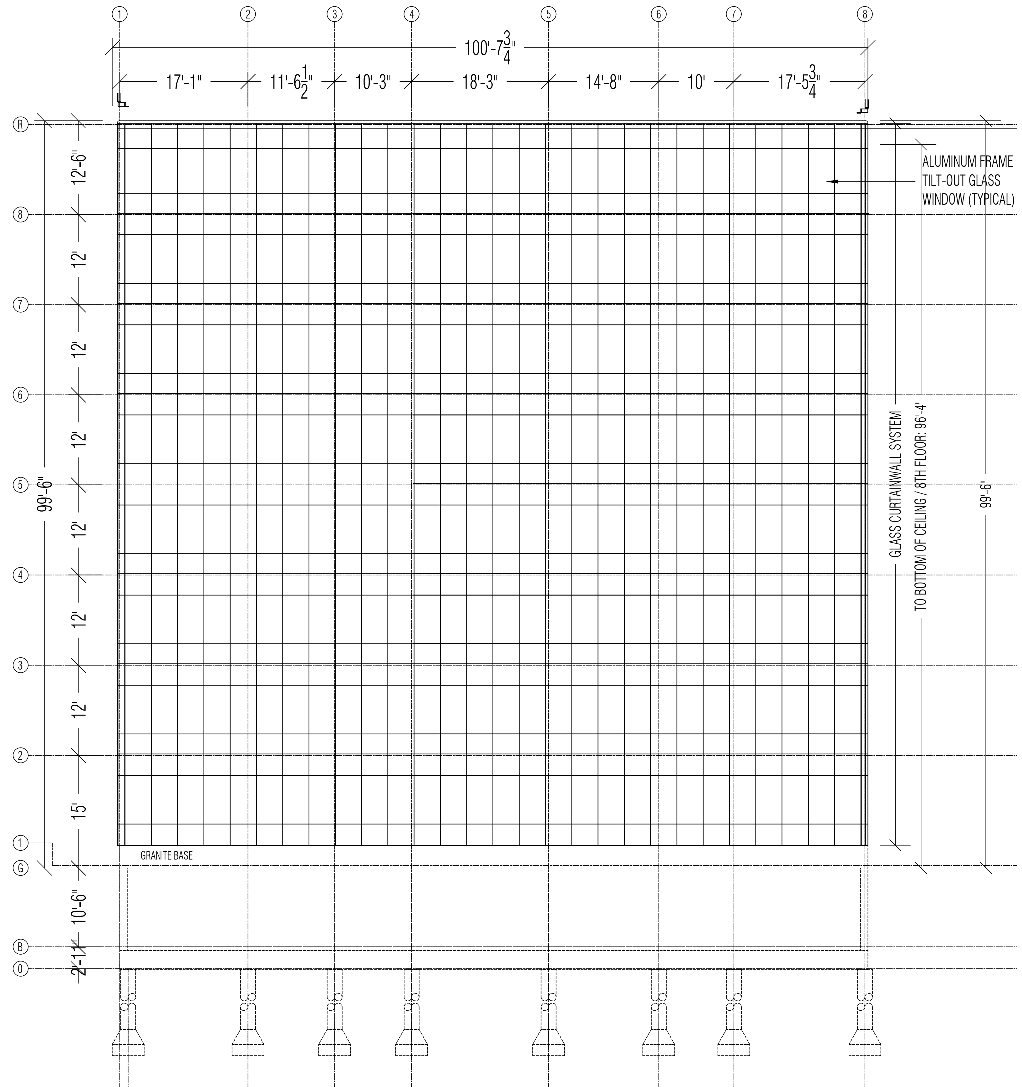
2 EAST ELEVATION Scale: 1/8" = 1'-0" 10 0 4 8 20
