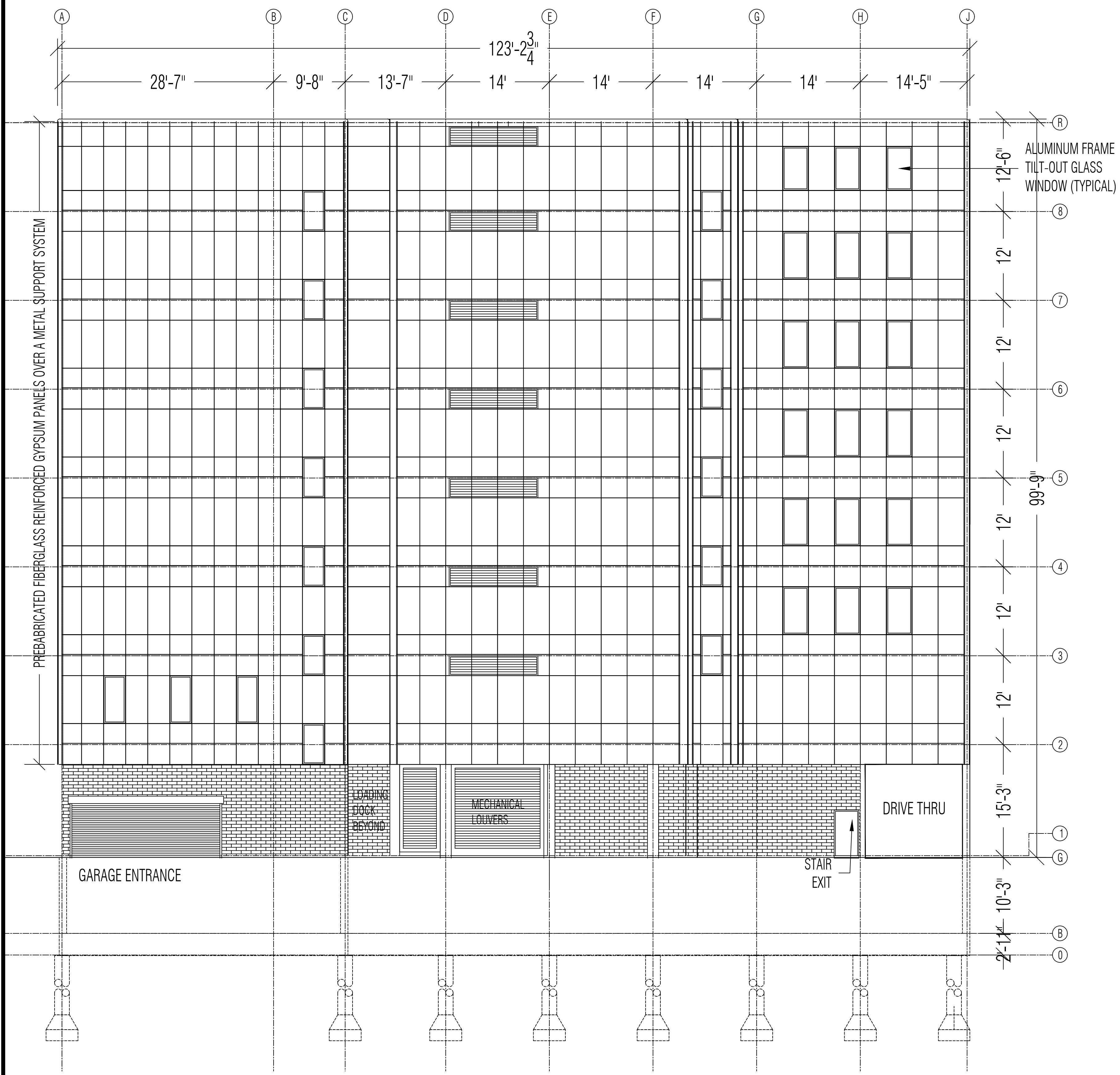
1 NORTH ELEVATION Scale: 1/8" = 1'-0"
